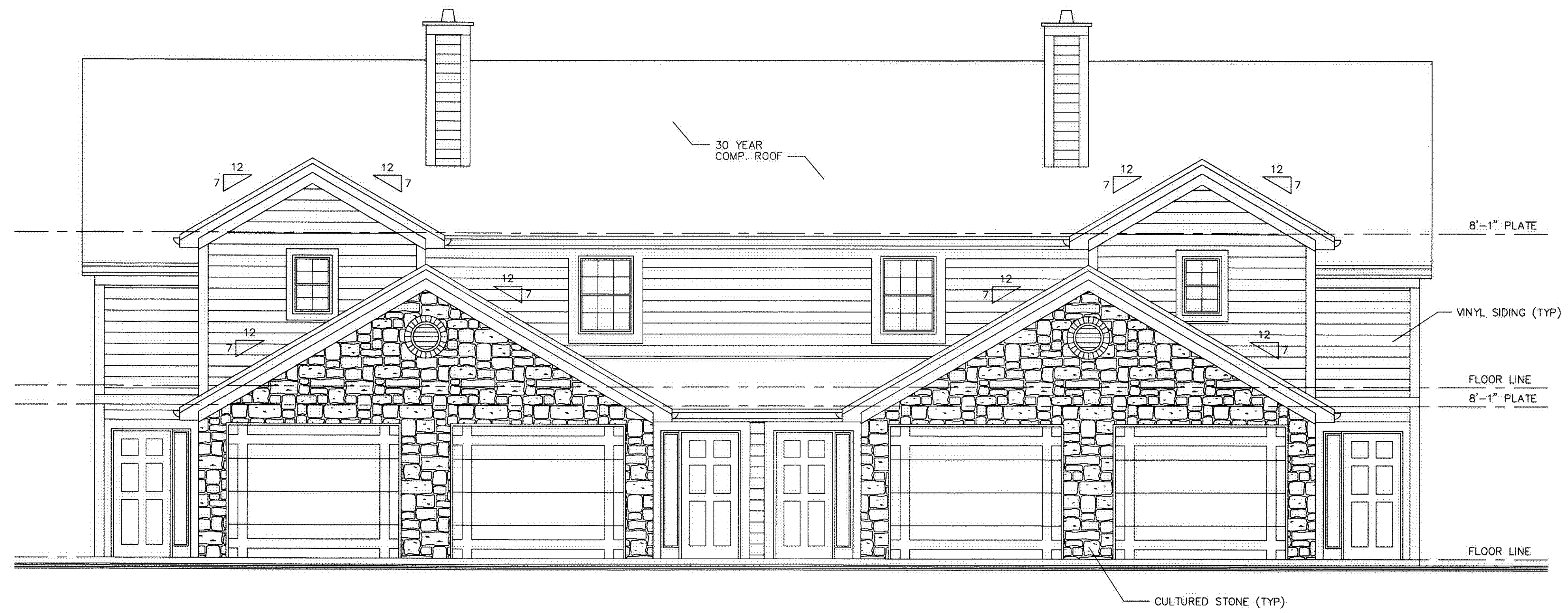
FRONT ELEVATION 06042EF SCALE: 1/4" = 1'-0"
